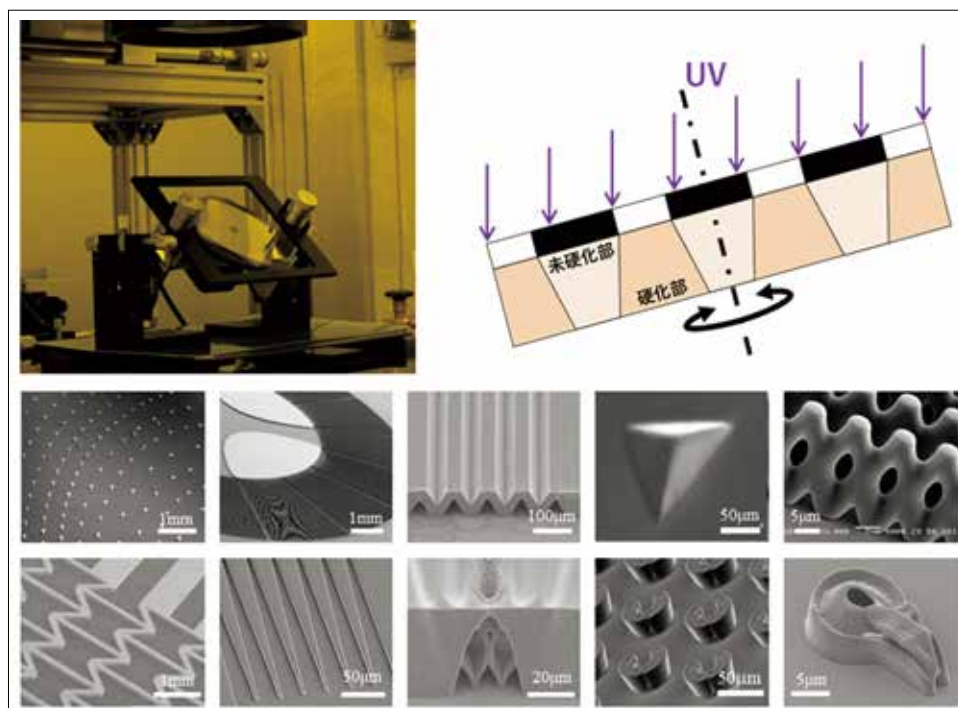
図2 3次元リソグラフィ法：
